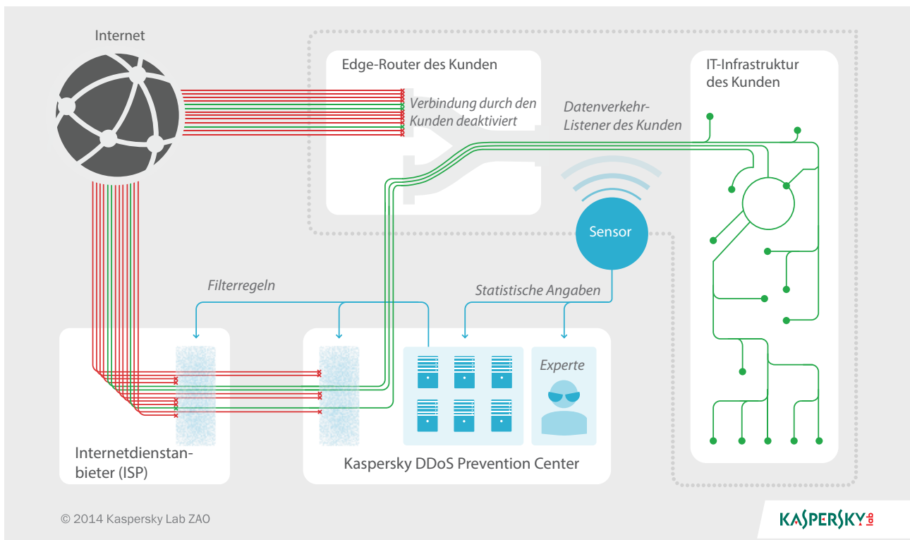
Abbildung 2: Kaspersky DDoS Protection-Ablaufdiagramm
